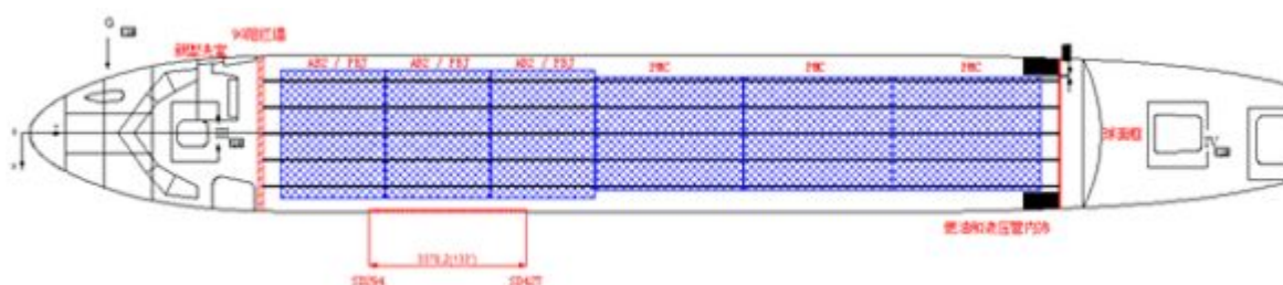
图 6 ARJ21-700CCF内部布局图 (7个PBJ) (共1张 第1张)
