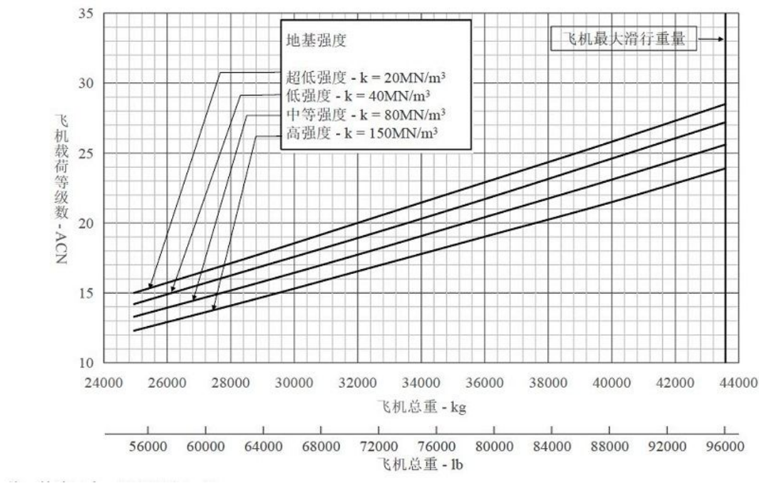
图 4 ARJ21-700ER硬道面ACN值 (共1张 第1张)
