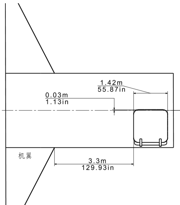
图 7 ARJ21-700 前货舱门间距 (共3张 第1张)
