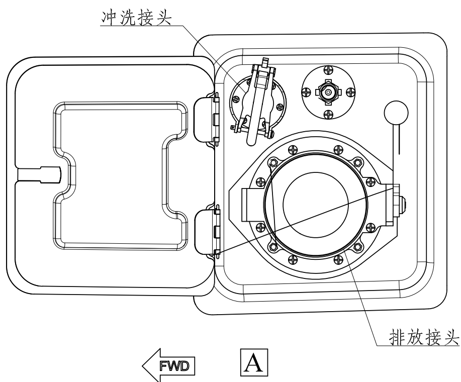
图 8 废水系统地面服务面板(共1张 第1张)
