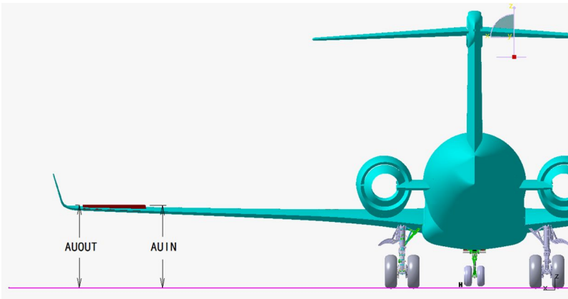
图 7 副翼升起状态离地高度示意图 (共1张 第1张)
