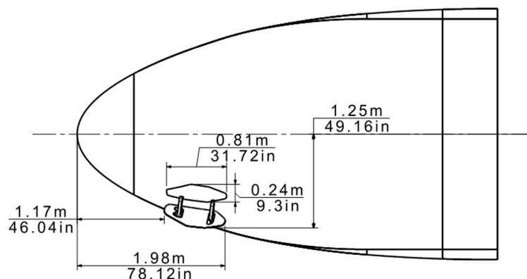
图 3 ARJ21-700应急门间距 (共3张 第3张)
