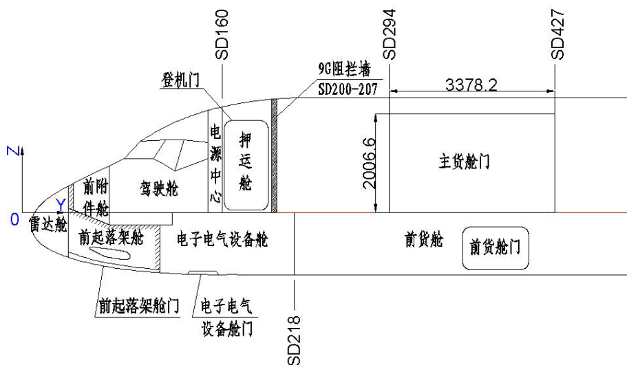
图 13 ARJ21-700CCF 主货舱门开口区域 (共1张 第1张)
