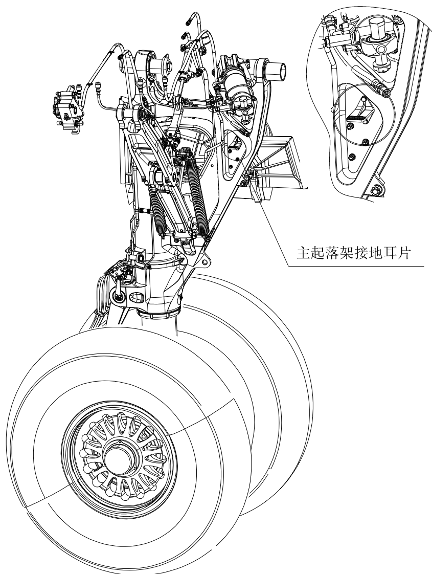
图 2 主起落架接地耳片 (共1张 第1张)
