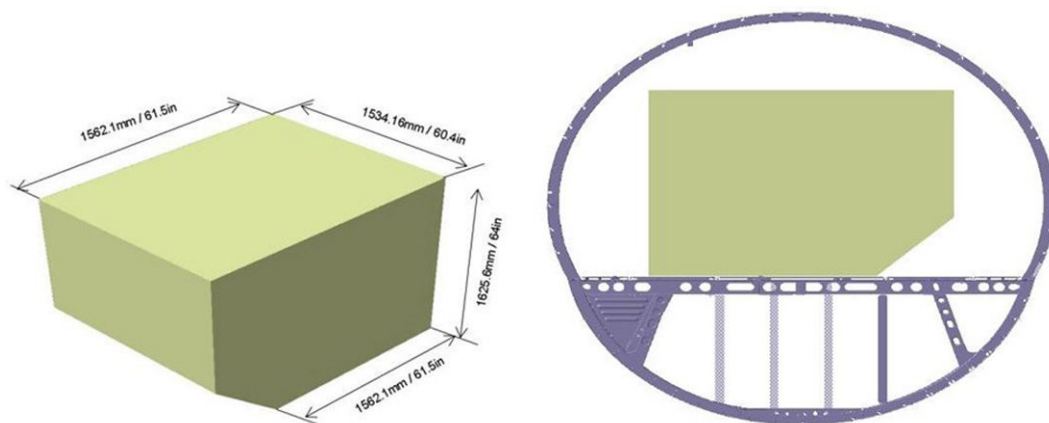
图 5 ARJ21-700CCF AB2集装箱/PBJ集装箱板在主货舱剖面布置情况(共1张 第1张)
