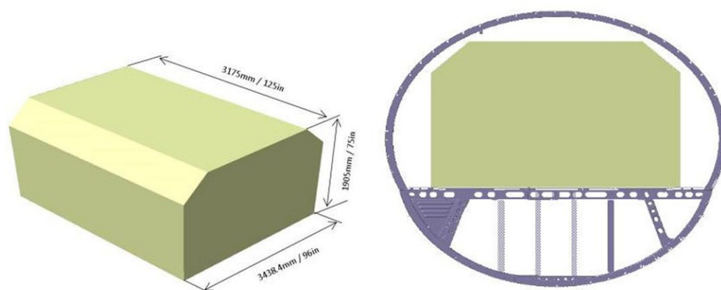
图 7 ARJ21-700CCF AAY集装箱/PAG集装箱板在主货舱剖面布置情况(共1张 第1张)
