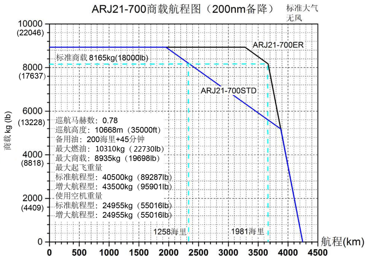
图 1 ARJ21-700商载航程图（全经济级/混合级）（共1张 第1张）
