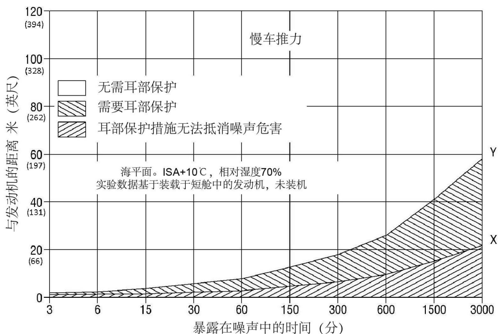
图 3 发动机噪音危害区域（起飞推力）（共1张 第1张）
