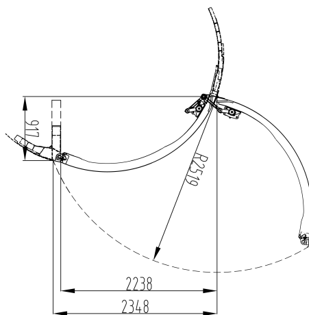
图 14 ARJ21-700CCF 主货舱门尺寸图 (共1张 第1张)
