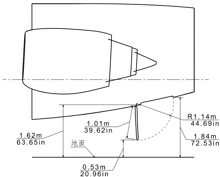
图 6 ARJ21-700 后附件舱门间距 (共2张 第1张)
