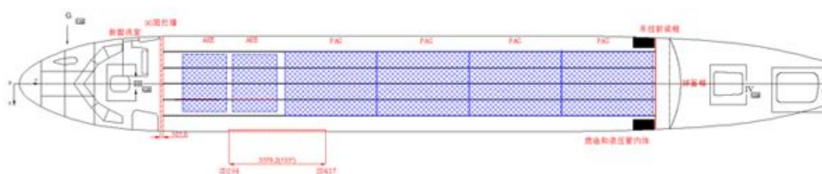
图 4 ARJ21-700CCF内部布局图 (2个AKE+4个PAG/AAY) (共1张 第1张)
