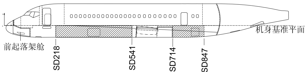
图 1 ARJ21-700 货舱及货舱门位置(共1张 第1张)
