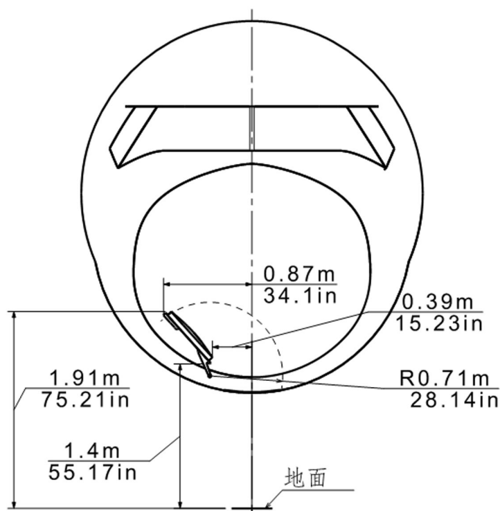
图 5 ARJ21-700 E-E舱门间距(共3张 第1张)
