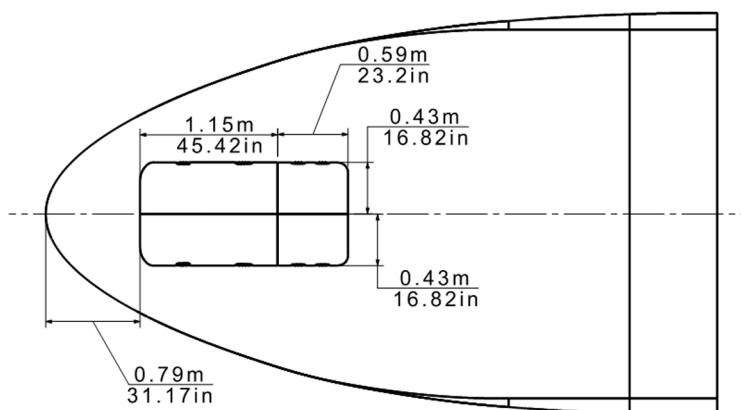
图 9 ARJ21-700 前起落架舱门间距 (共3张 第1张)
