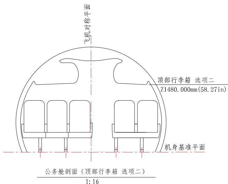
图 2 ARJ21-700 78座混合型客舱截面 (共3张 第2张)
