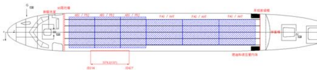
图 8 ARJ21-700CCF内部布局图（3个AB2/PBJ+3个PAG/AAY）（共1张 第1张）
