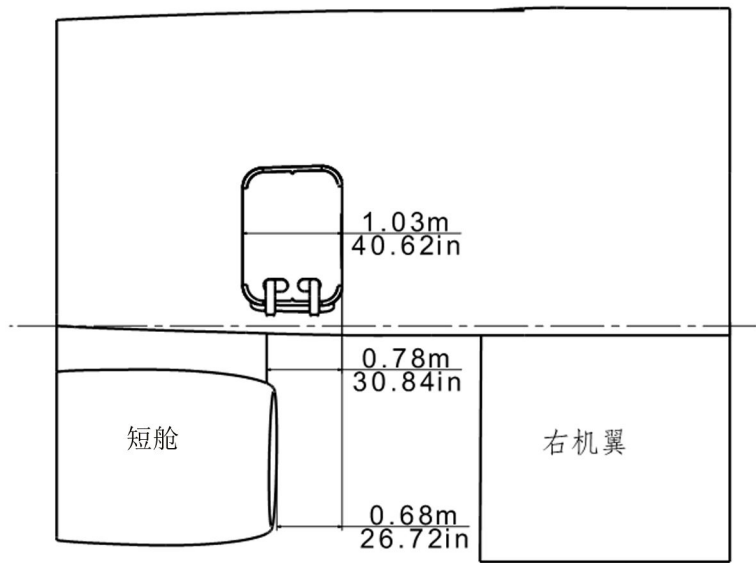
图 8 ARJ21-700 后货舱门间距(共3张 第2张)
