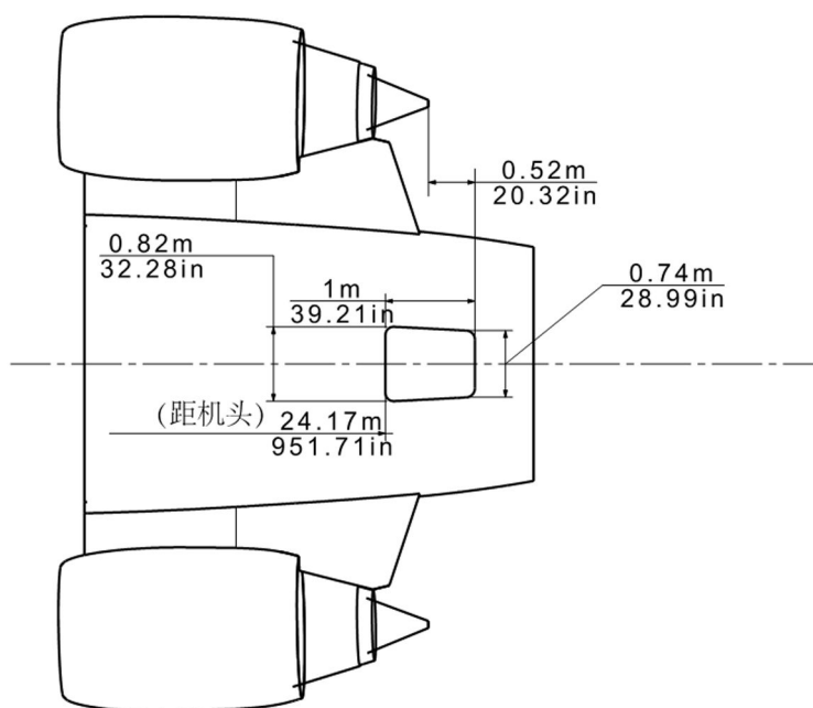
图 6 ARJ21-700 后附件舱门间距 (共2张 第1张)
