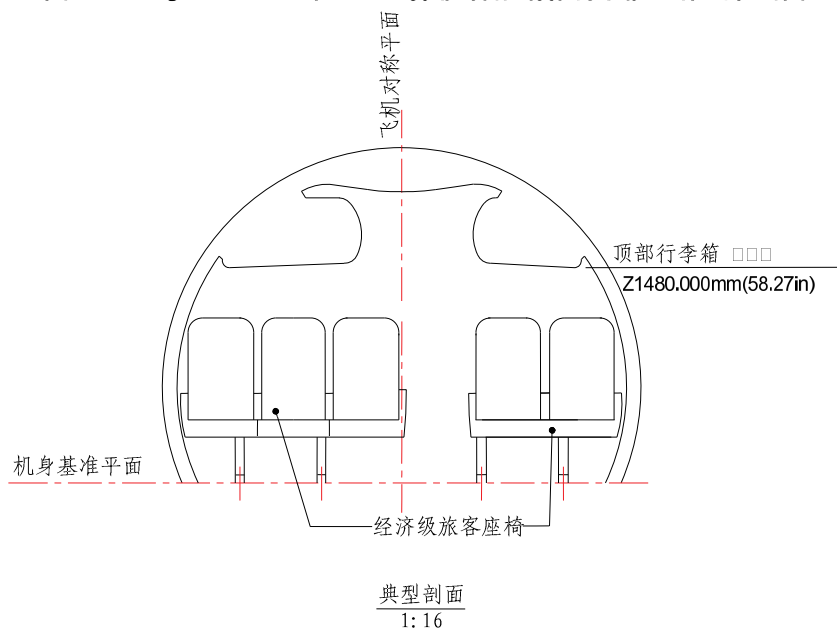
图 1 ARJ21-700 90座全经济级客舱截面图(共3张 第1张)
