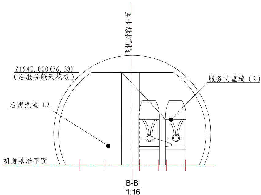
图 2 ARJ21-700 78座混合型客舱截面 (共3张 第2张)
