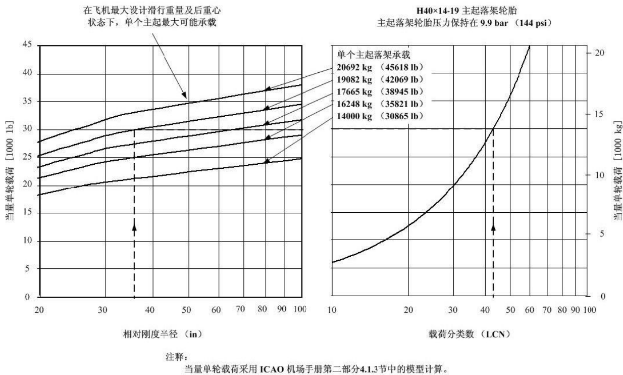
图 2 硬道面载荷等级值的换算(共1张 第1张)
