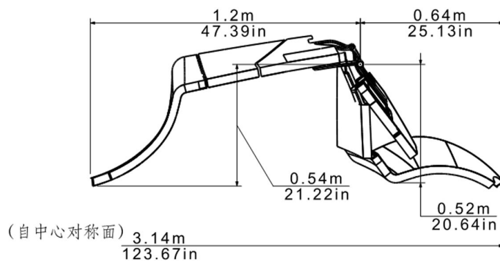
图 10 ARJ21-700 主起落架舱门间距 (共3张 第2张)
