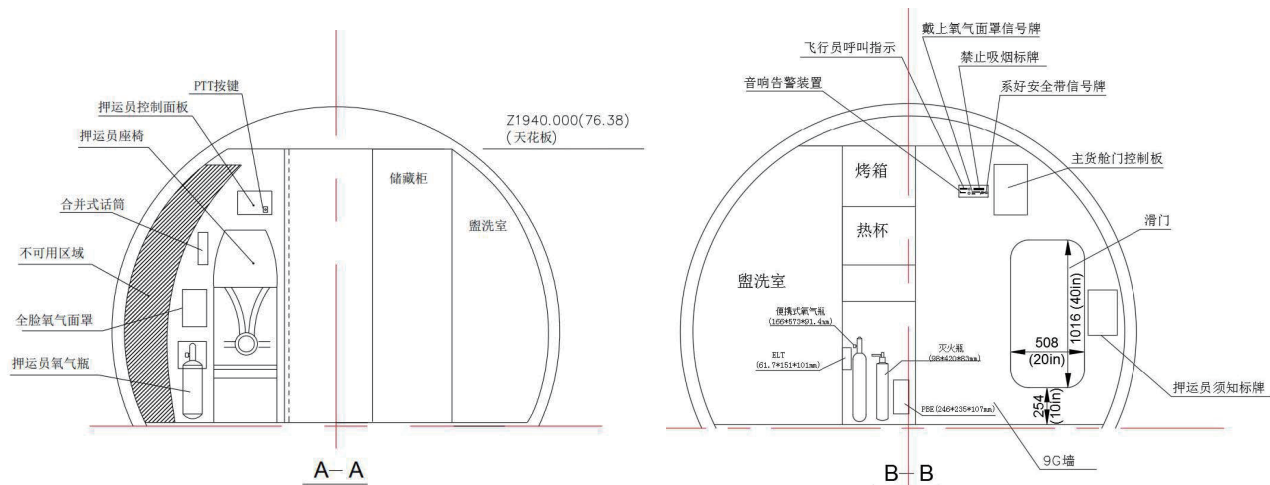
图 5 ARJ21-700CCF 押韵舱前视图及后视图 (共1张 第1张)
