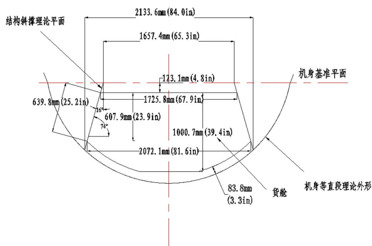
图 1 ARJ21-700 货舱及货舱门位置(共1张 第1张)
