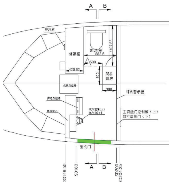
图 4 ARJ21-700CCF 押韵舱俯视图(共1张 第1张)
