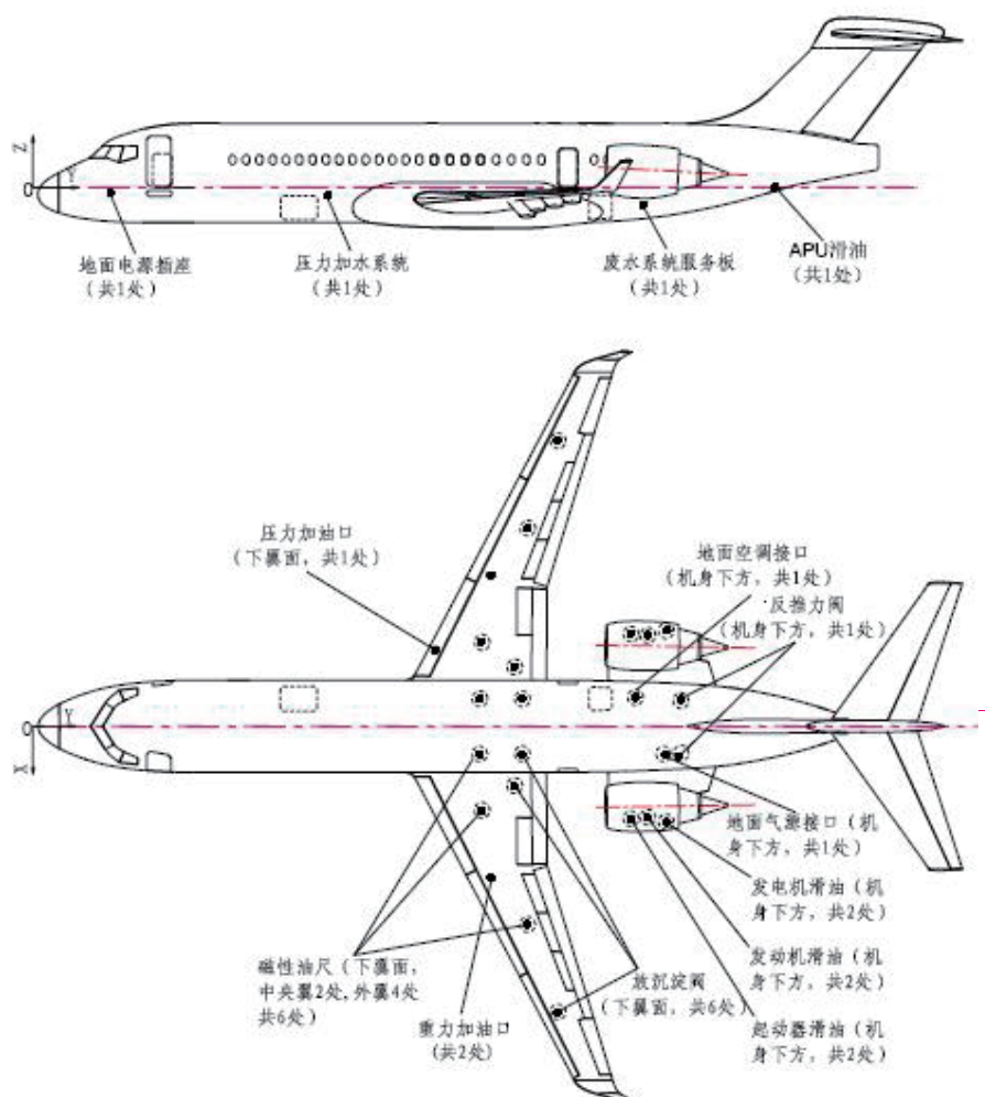
图 1 地面保养服务点位置(共1张 第1张)
