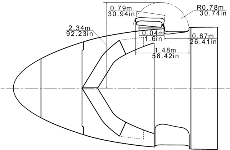
图 1 ARJ21-700登机门间距(共3张 第3张)
