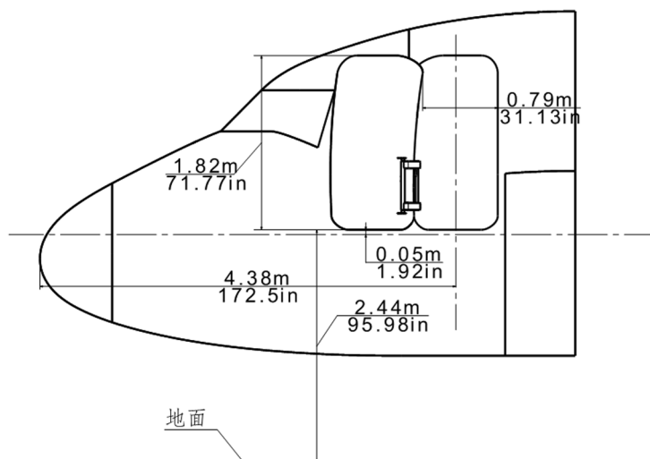
图 1 ARJ21-700登机门间距 (共3张 第1张)
