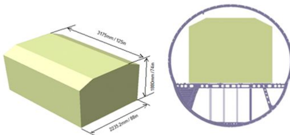
图 7 ARJ21-700CCF AAY集装箱/PAG集装箱板在主货舱剖面布置情况(共1张 第1张)
